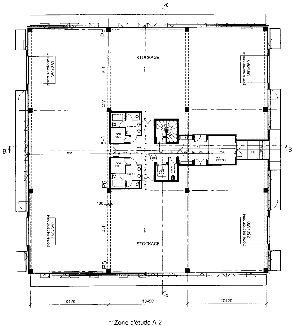
REZ DE CHAUSSEE Echelle : 1/200
