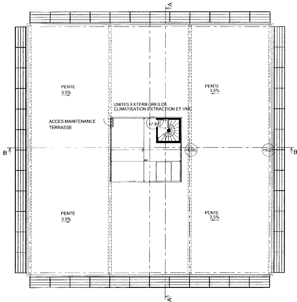
NIVEAU 2 - TOITURE-TERRASSE
