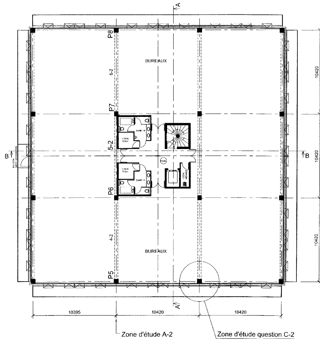
NIVEAU 1 Echelle : 1/200
